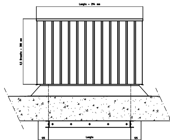
Zijaanzicht
