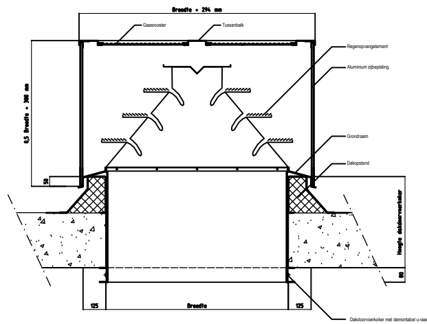
Doorsnede
