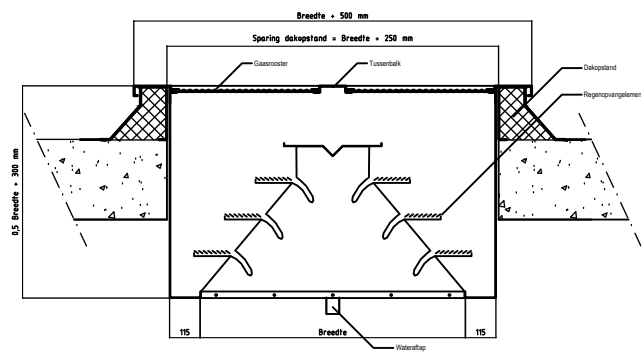
Doorsnede
