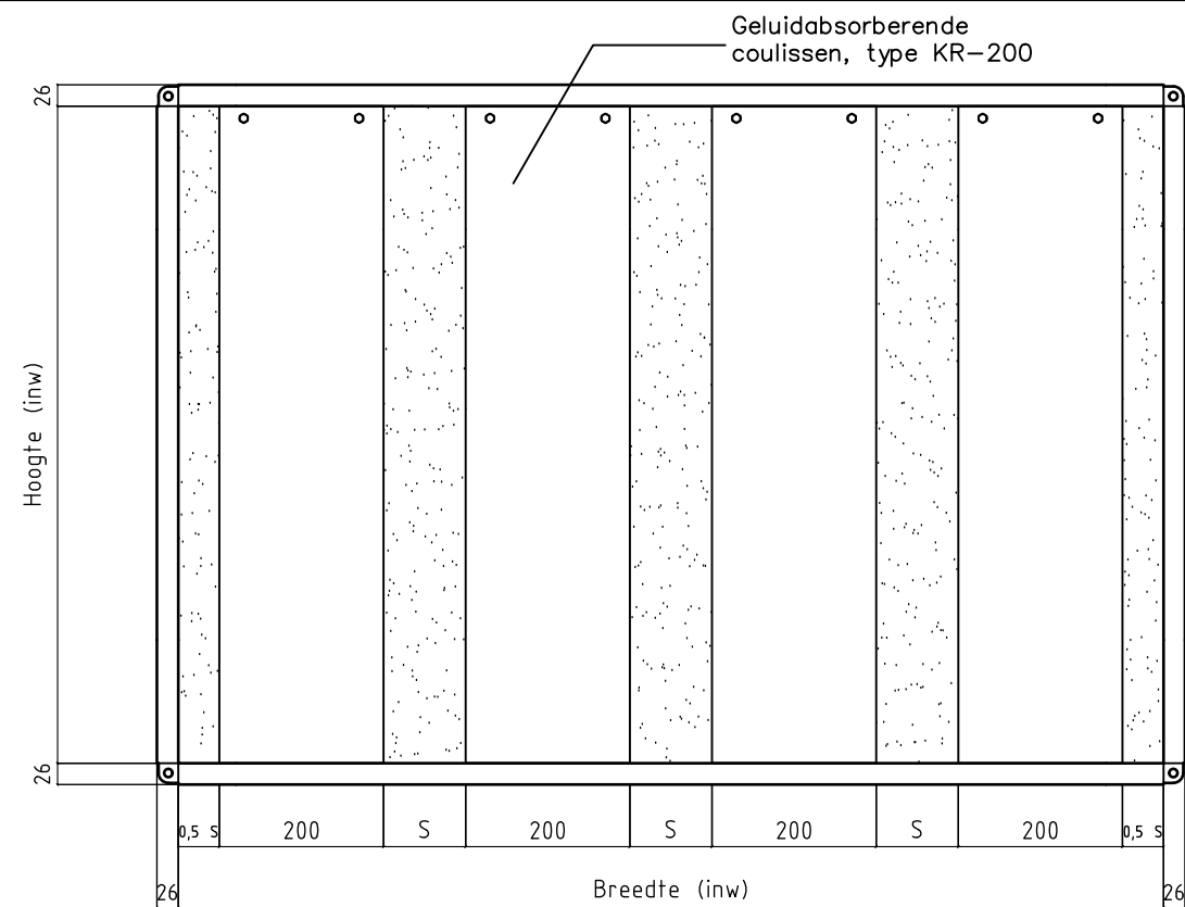
Vooraanzicht
