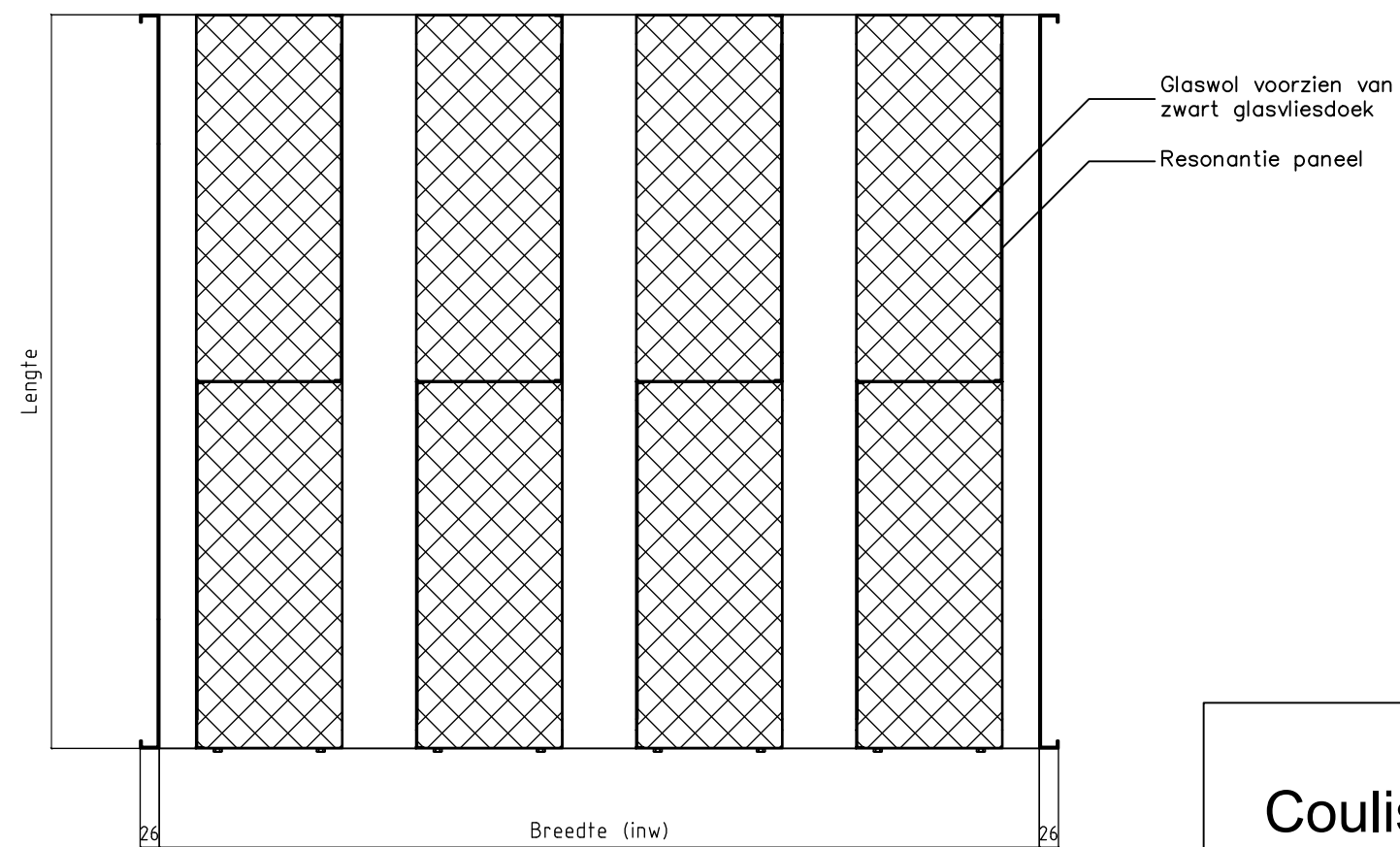
Doorsnede
