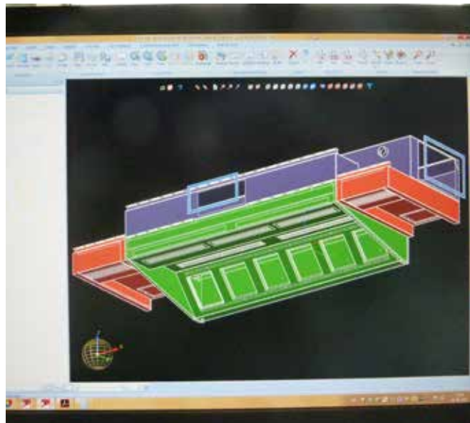
3D-model custom build afzuigkap t.b.v. een luxe jacht.
