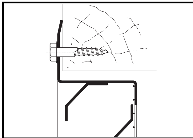
Figuur 2a: Type BV-70 in houten stelkozijn
