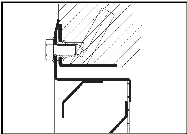
Figuur 1a: Type BV-70 met inmettselraam IR
