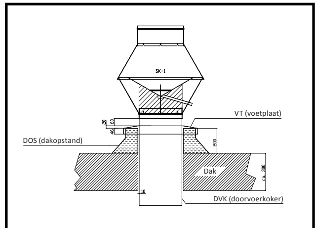
Figuur 6: SK-1 + DVK + voet + DOS
