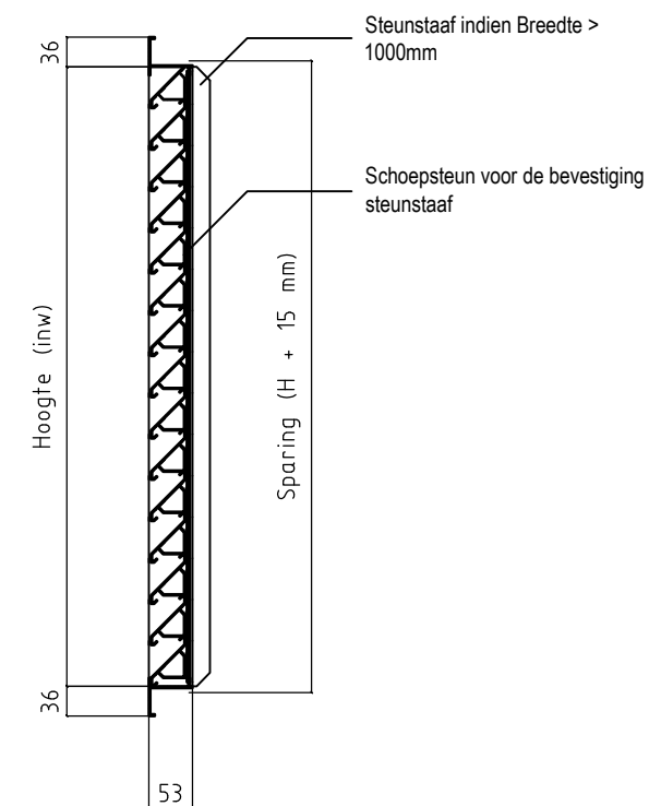
Doorsnede
