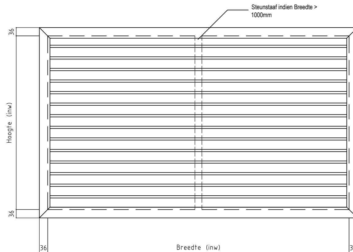
Vooraanzicht
