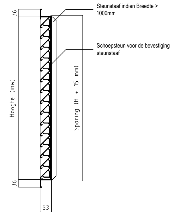
Doorsnede
