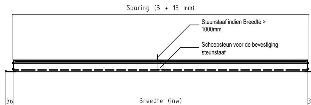
Doorsnede
