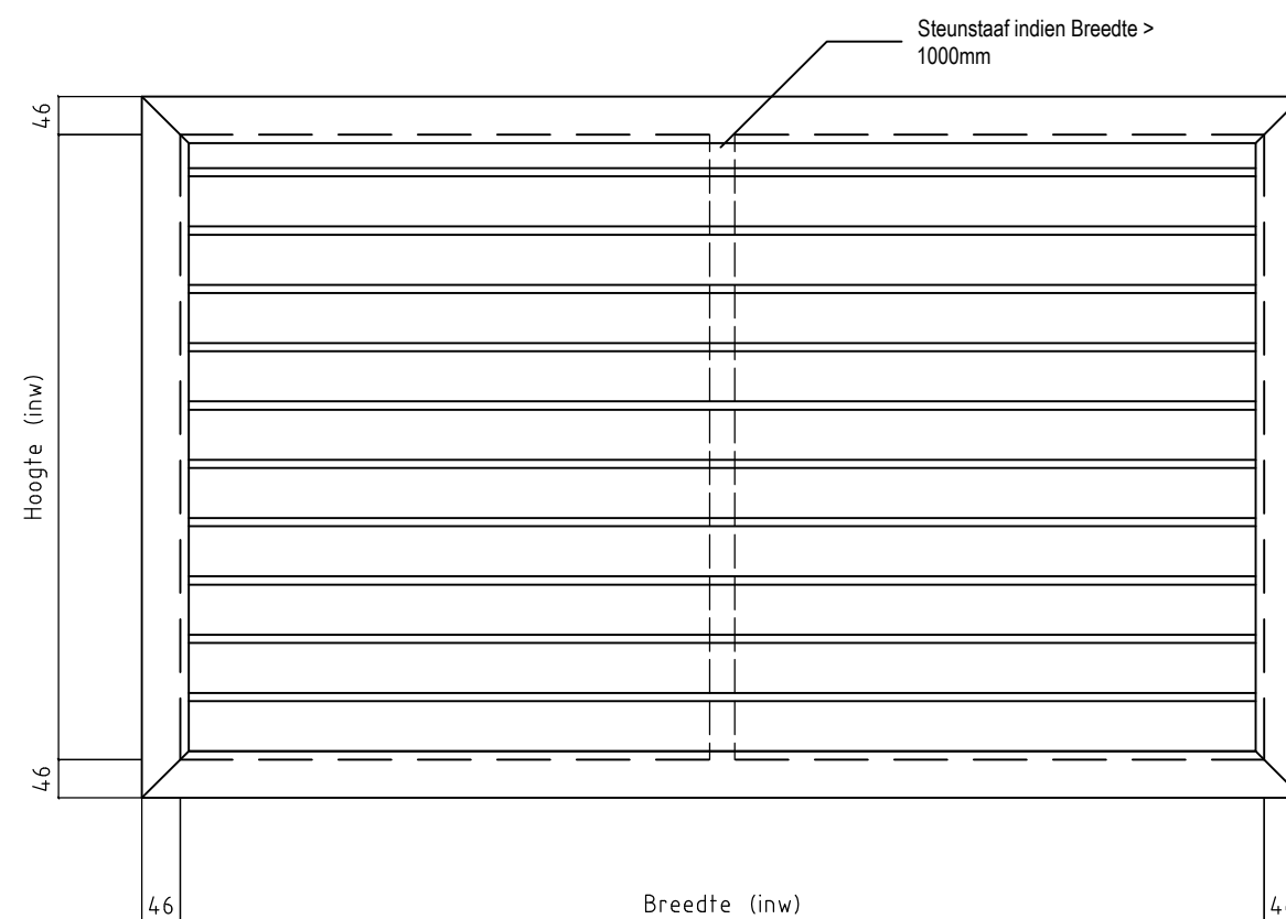
Vooraanzicht
