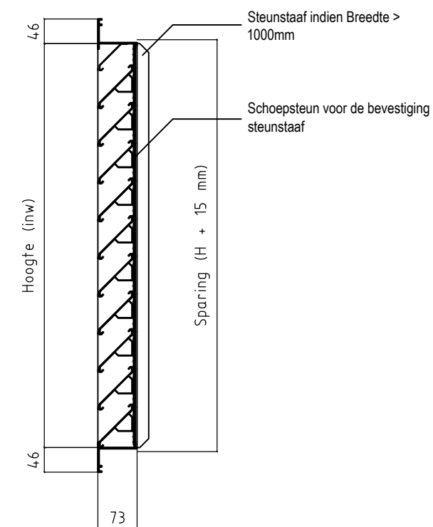
Doorsnede
