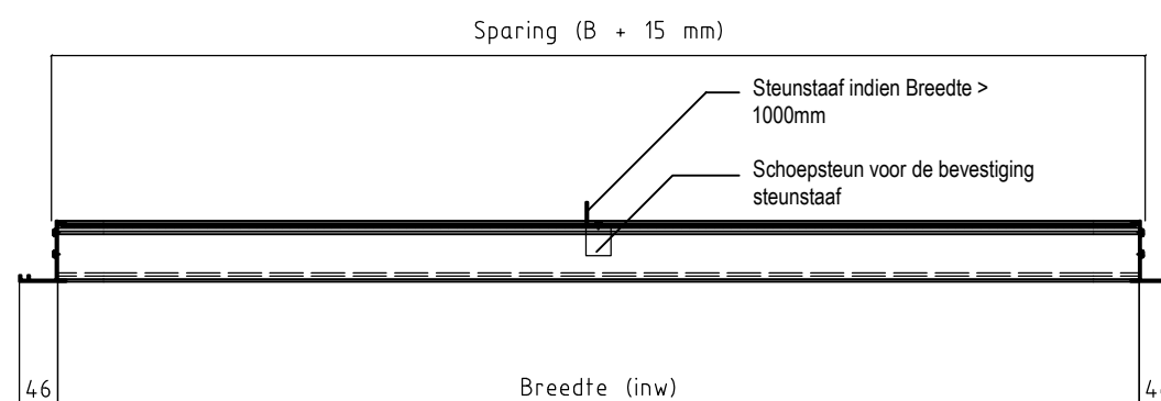
Doorsnede
