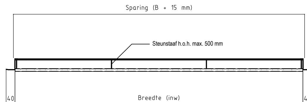
Doorsnede
