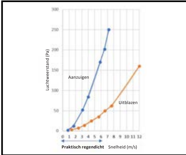
Luchtweerstand type SK-1
