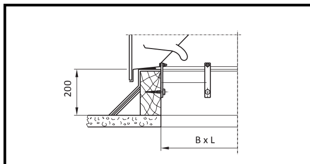
Figure 2 : Fixation à l'intérieur du lanterneau (par des tiers).
