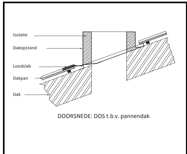
Figuur 2: Schuin pannendak.
