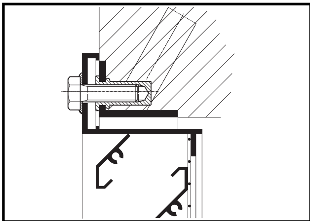
Figuur 1a: Type BA-70 met IR-A
