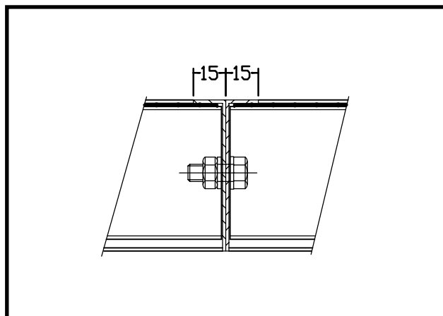
Figuur 4: Een breedtedeling
