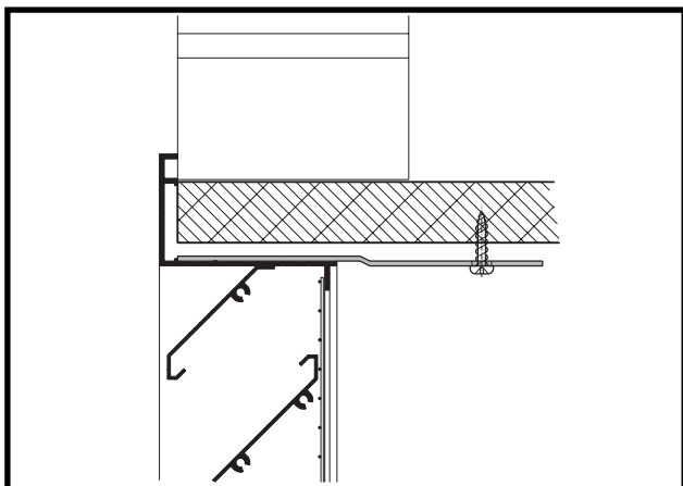
Figuur 1b: Bevestiging middels strippen aan achterzijde
