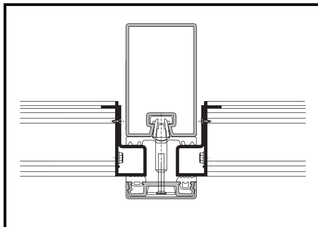
Figuur 2b: Bevestiging in gevel- / raamprofiel
