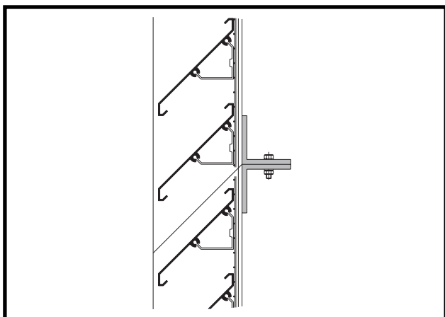
Figuur 3: Een hoogtedeling
