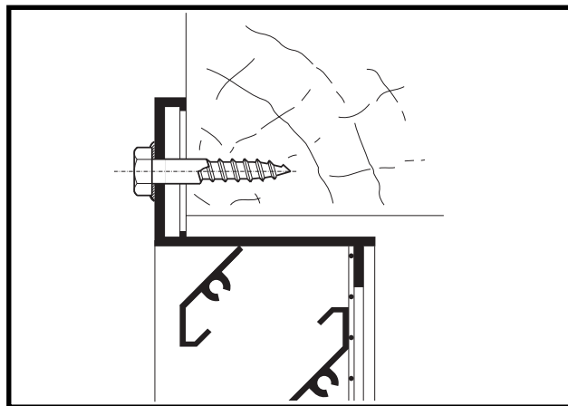
Figuur 2a: Type BA-70 in houten stelkozijn
